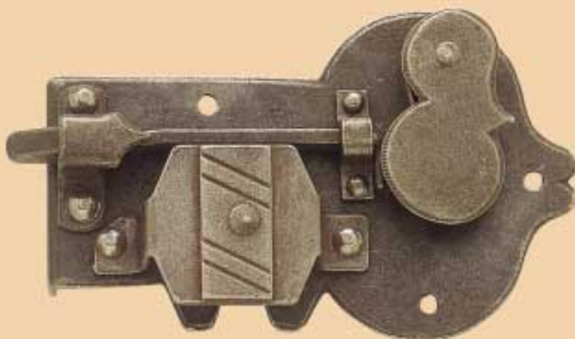
Réf : 375-20 axe : 35/40/50/55/60 Dt ou G
