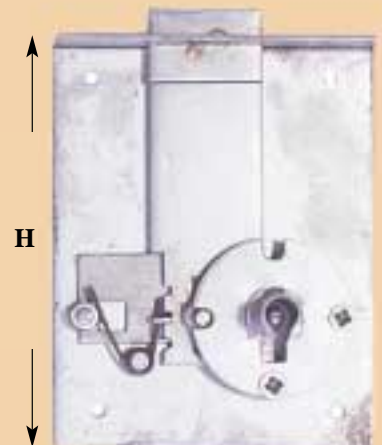
26BIS Serrure à entailler
